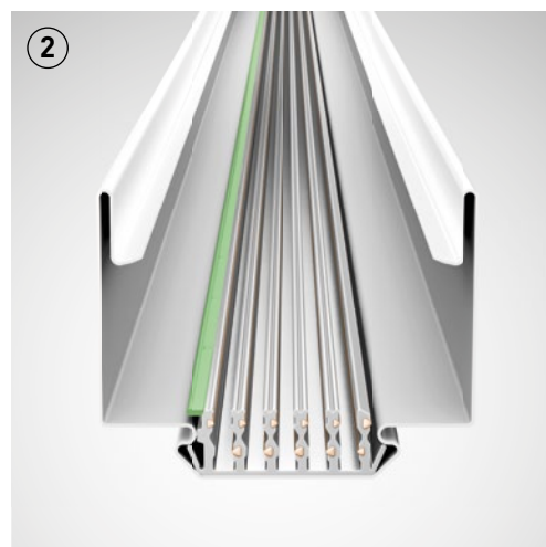
11-aderig stroomvoerend profiel 5 \times 2,5 \text{ mm}^2 + 6 \times 1,5 \text{ mm}^2 3 afzonderlijke stroomkringen 2-stuurleidingen voor DALI-sigitaal 2 onafhankelijke stroomkringen voor de noodverlichting
