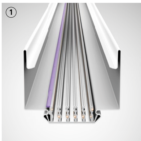
7-aderig stroomvoerend profiel 5 \times 2,5 \text{ mm}^2 + 2 \times 1,5 \text{ mm}^2 3 afzonderlijke stroomkringen 2-stuurleidingen voor DALI-sigitaal
