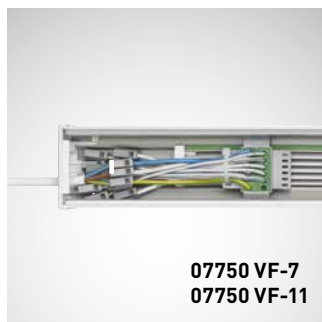
Connecteur à 7 ou 11 conducteurs pour connexion électrique, flexible
