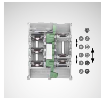
Connettore Flex, a 11 poli*
