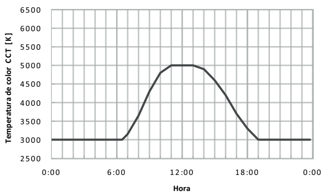
Figura 2.1: La curva HCL de TRILUX
