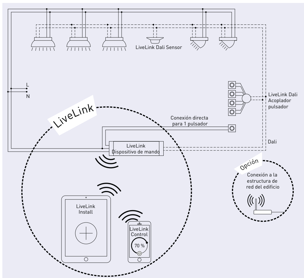
Figura 1.1: Resumen de los componentes del sistema LiveLink
